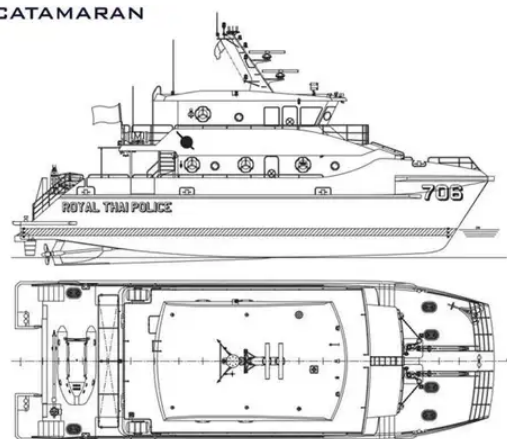
23M. CATAMARAN
